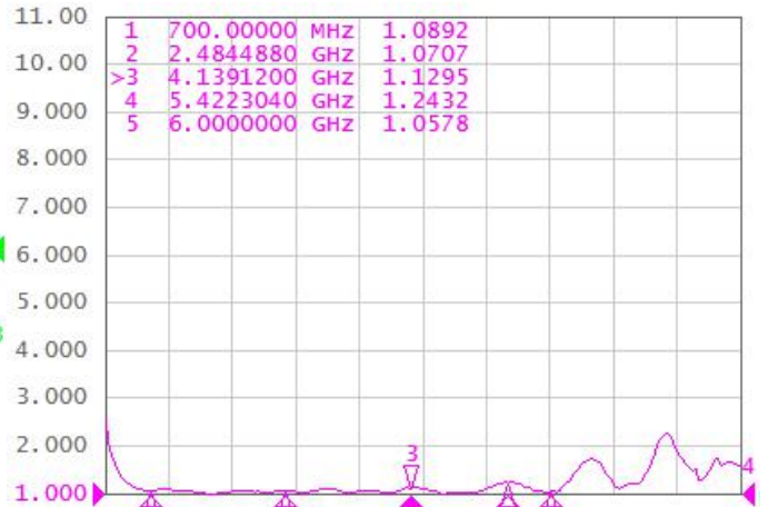
图4 输出端驻波测试结果
