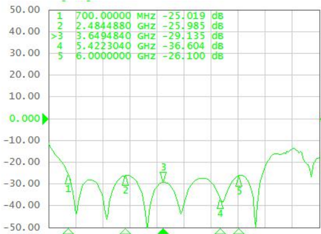
图3 隔离度测试结果
