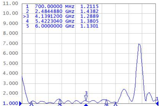
图2 输入端驻波测试结果
